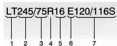
Llantas para camiones ligeros (LT-Métrico)
